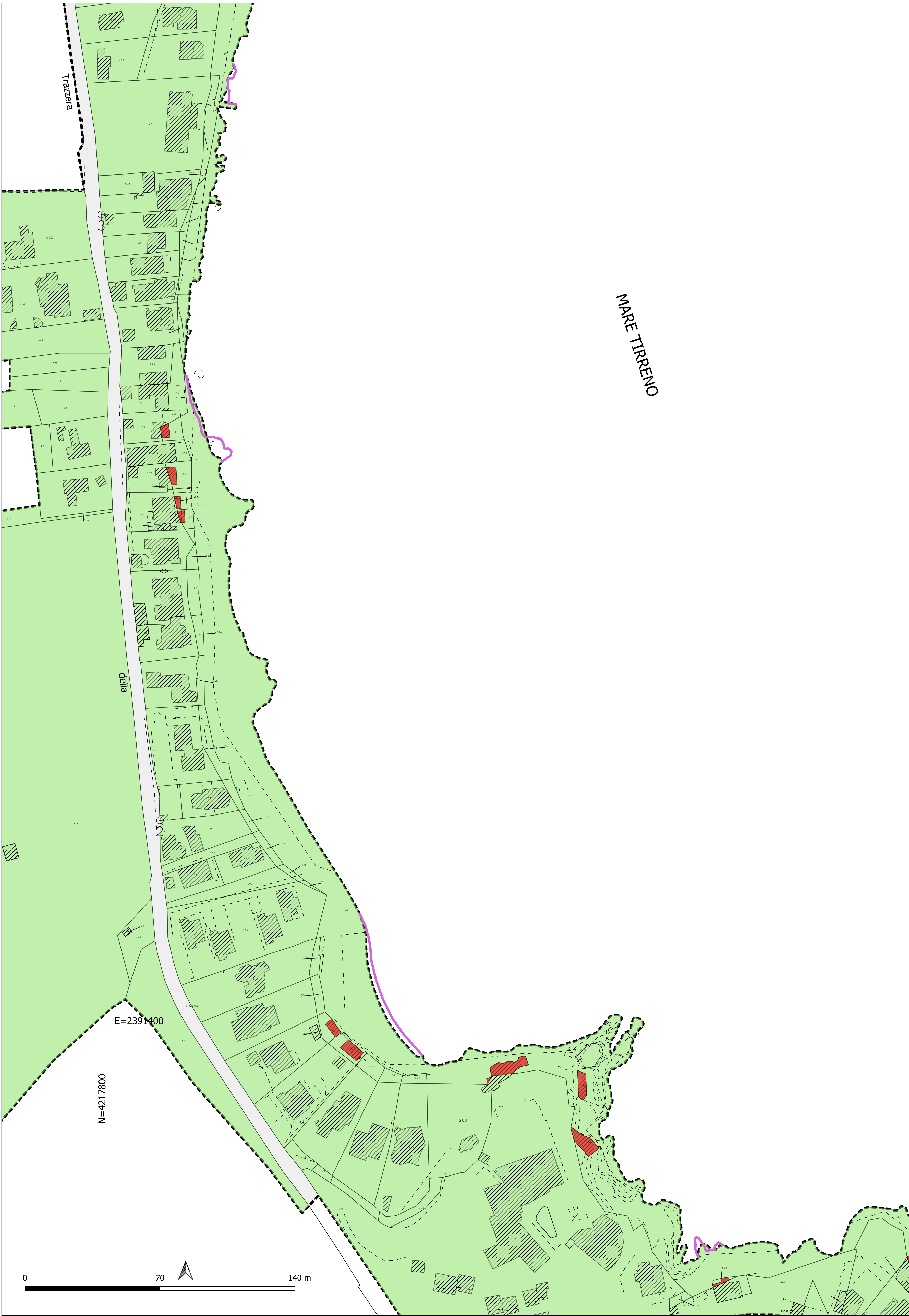
AREA 2 LINEE REV E FABBRICATI RICADENTI IN AREA DEMANIALI SCALA 1: 1.000
